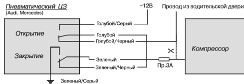
Пневматический ЦЗ (Audi, Mercedes)
