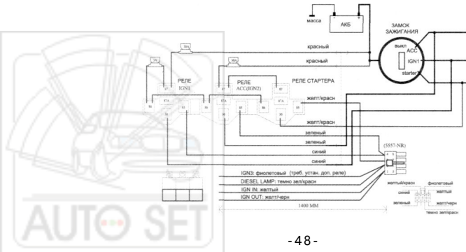
СХЕМА СОЕДИНЕНИЙ В РЕЖИМЕ АВТОЗАПУСКА БЕЗ ИСПОЛЬЗОВАНИЯ ТУРБОТАЙМЕРА
