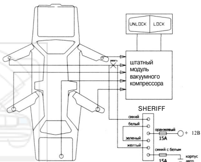
СХЕМА УПРАВЛЕНИЯ ВАКУУМНЫМИ СИСТЕМАМИ Mercedes-Benz, Audi
