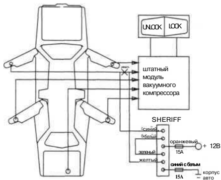
СХЕМА УПРАВЛЕНИЯ ВАКУУМНЫМИ СИСТЕМАМИ Mercedes-Banz, Audi
