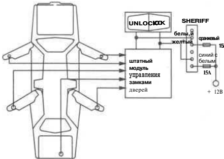
Положительный триггер (большинство легковых автомобилей «Дженерал Моторс»)
