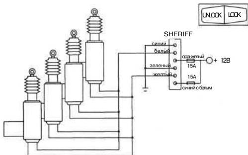
СХЕМА УПРАВЛЕНИЯ ДОПОЛНИТЕЛЬНЫМИ ЭЛЕКТРОПРОВОДАМИ
