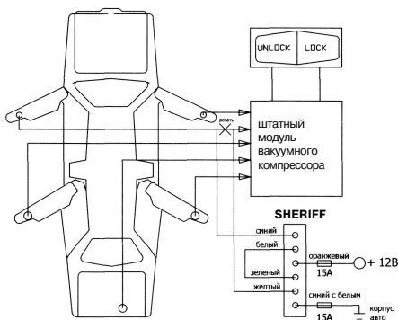
СХЕМА УПРАВЛЕНИЯ ДОПОЛНИТЕЛЬНЫМИ ЭЛЕКТРОПРОВОДАМИ
