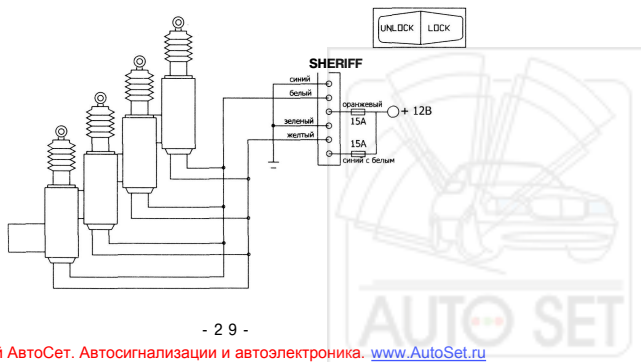
СХЕМА УПРАВЛЕНИЯ ДОПОЛНИТЕЛЬНЫМИ ЭЛЕКТРОПРОВОДАМИ
